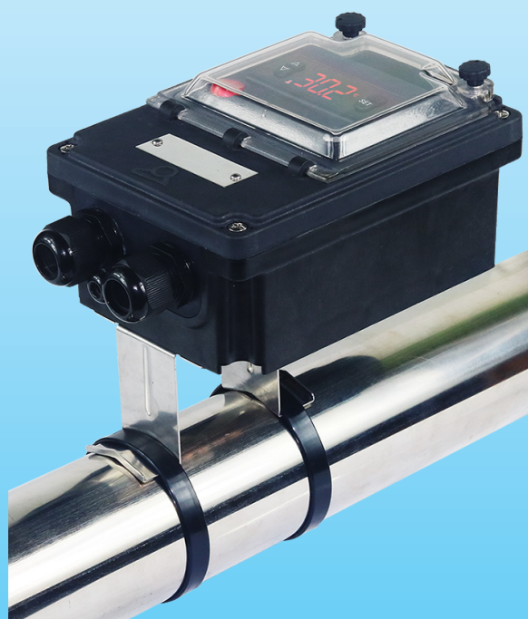
Exemple de montage avec l'option platine arrière de montage sur tube vertical
