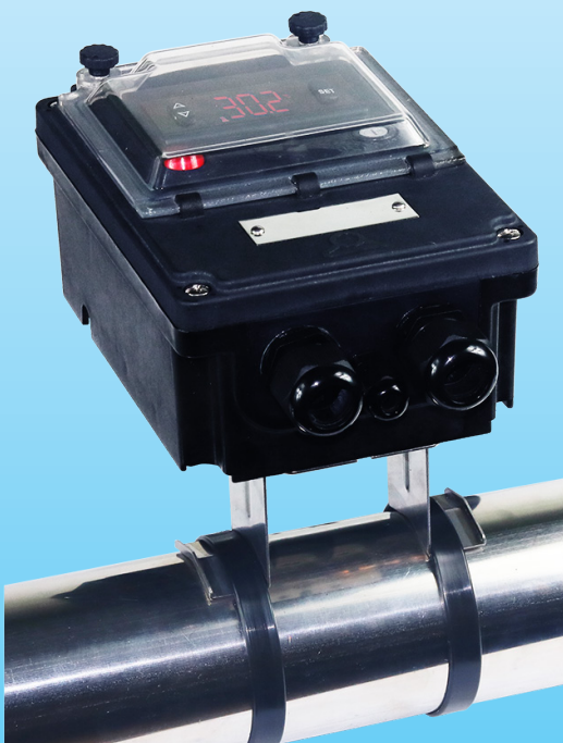
Exemple de montage avec l'option platine arrière de montage sur tube horizontal
