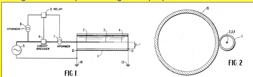
Extrait d'un brevet de Masao Ando de 1968, pour la Chisso corporation à Osaka, décrivant le réchauffage de pipelines par une tube chauffant à courant de Foucault.
